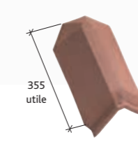
About d'arêtier angulaire à emboîtement Réf. 859
