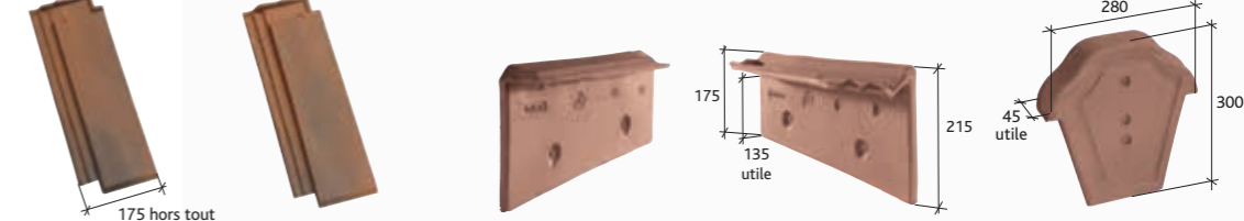
1/2 tuile Diamant gauche Réf.219.02 1/2 tuile Diamant droite Réf.219.01 Rive individuelle gauche nouveau modèle Diamant (2,7 par ml) Réf. 219.44 Rive individuelle droite nouveau modèle Diamant (2,7 par ml) Réf. 219.43 Fronton pour faîtière losangée à recouvrement Réf. 809
