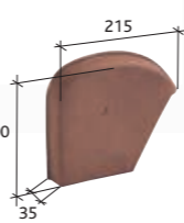
Fronton gauche pour faîtière Shed Réf. 806 (2)
