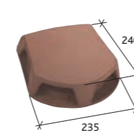
Lanterne bi-section Ø 126 utile et Ø 160 utile (Section d'aération : 130 cm 2 ) (conforme VMC) Réf. 1000
