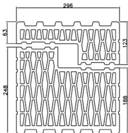
Feuillure 12 R30
