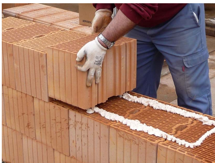
Figure 11– Pose des briques en partie courante.
