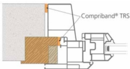
Croquis 18 : Mise en œuvre en rénovation
