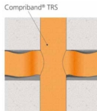
Croquis 11 : Raccords en croix
