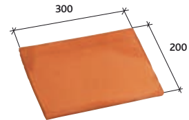
Bardelis droit 20 x 30 (2) Réf. 1056
