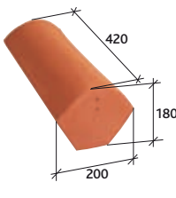
About de faîtière à sec (2) grande ouverture Réf. 826 petite ouverture Réf. 827
