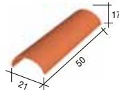
1 CL Tuile canal languedocienne 2,5 au ml - 2,6 kg
