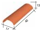
1 CV Tuile canal vendéenne 3,4 au ml - 1,5 kg
