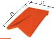
611 P17 Tuile chatière « passe-barre » 35 cm 2 - 1,5 kg
