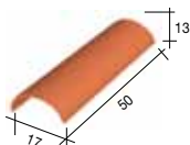
1 CG Tuile canal girondine 2,5 au ml - 1,9 kg
