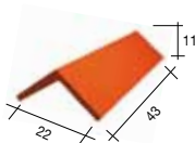
33 XGP Faîtière angulaire 2,9 au ml - 3,2 kg
