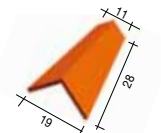
432 XGP Arêtier cornier angulaire (type nord) 10 au ml - 1,6 kg
