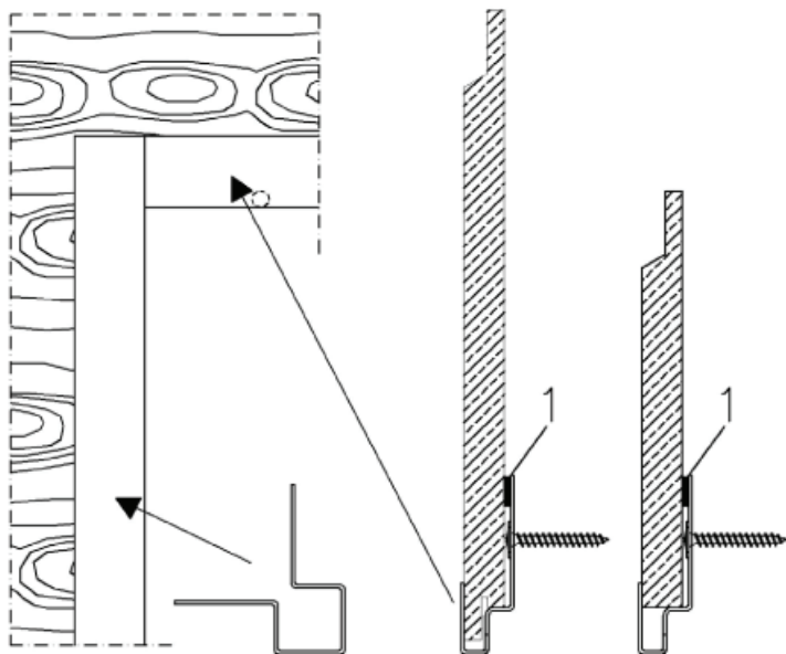
Profil d'angle extérieur Cédral Click
