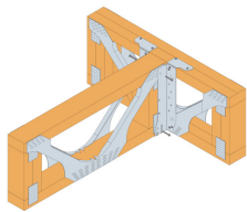
Fixation sur une poutre métallique ajourée
