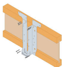
Fixation par les brides latérales sur un support poutre en I
