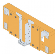
Fixation par les brides supérieures sur une poutre métallique ajourée avec renfort bois
