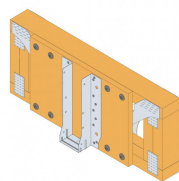
Fixation par les brides latérales sur une poutre métallique ajourée avec renfort bois
