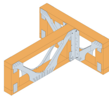
Fixation sur une poutre métallique ajourée
