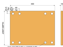
Dimension des blocs de renforts bois
