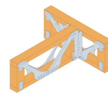
Fixation sur une poutre métallique ajourée
