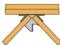
2 arêtiers sans empannon
