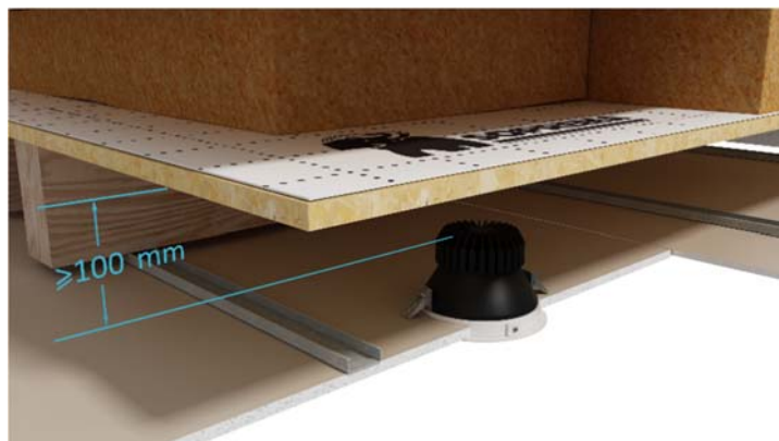
Figure 3. Spot encastré dans un plénum
