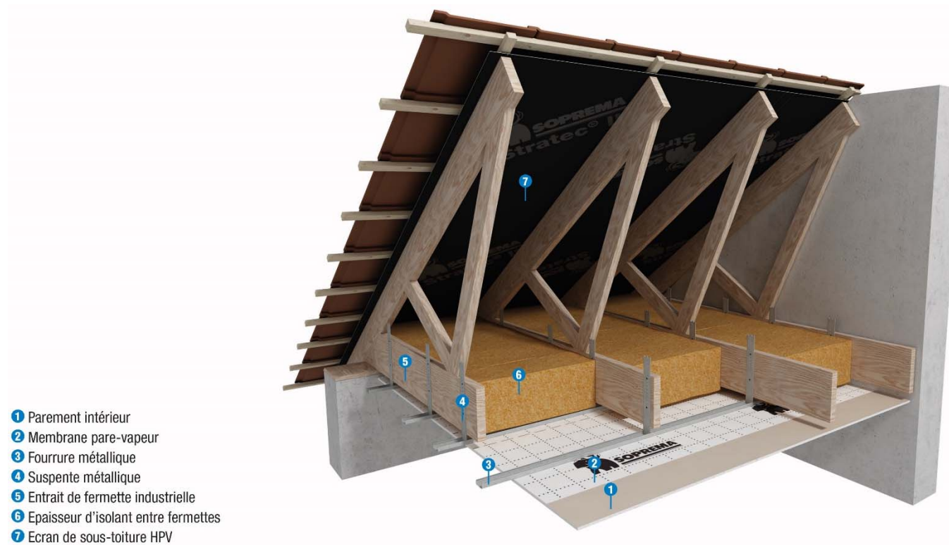
Figure 5. Mise en œuvre des produits « PAVAFLEX® CONFORT » et « PAVAFLEX® CONFORT 36 » entre solives, ou entre pieds de fermettes industrielles dans le cas d'un comble perdu ventilé
