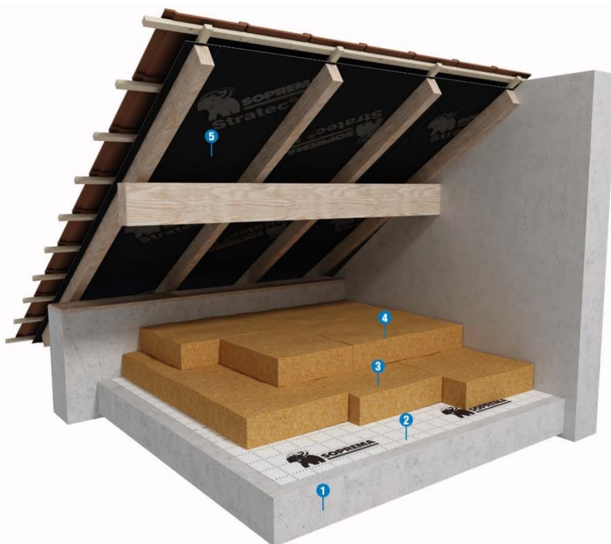
Figure 7 : Mise en œuvre des produits « PAVAFLEX® CONFORT » et « PAVAFLEX® CONFORT 36 » dans le cas d'un comble perdu ventilé sur plancher béton.
