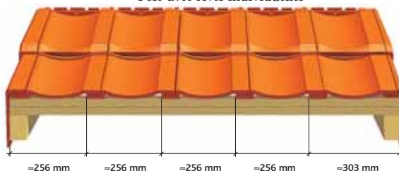
Pose avec rives individuelles
