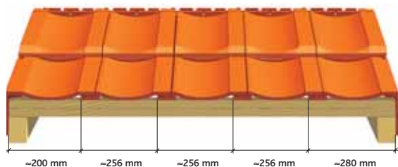
Pose avec tuiles de rives à rabat
