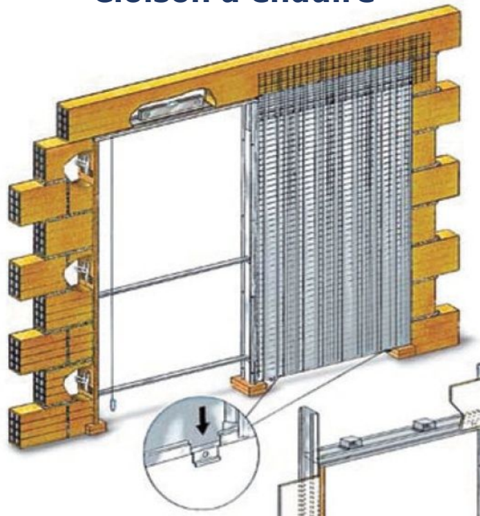
Cloison à enduire
