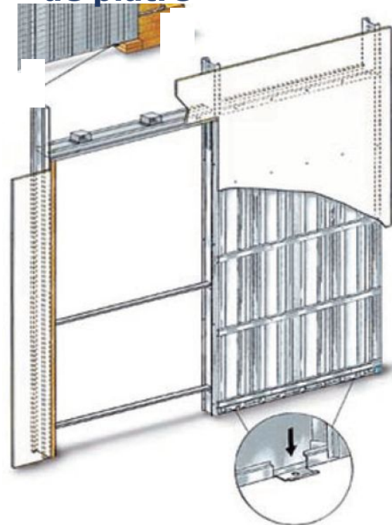
Cloison en plaques de plâtre
