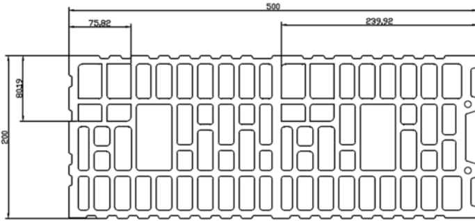
Figure 11 – Briques Tableau/Feuille
