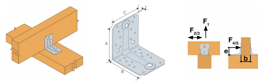
Fixation bois/bois
