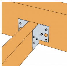
Fixation de pannes sur support bois
