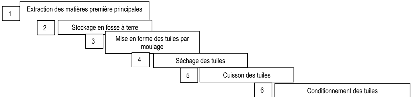
Schéma décrivant le procédé classique de fabrication des tuiles
