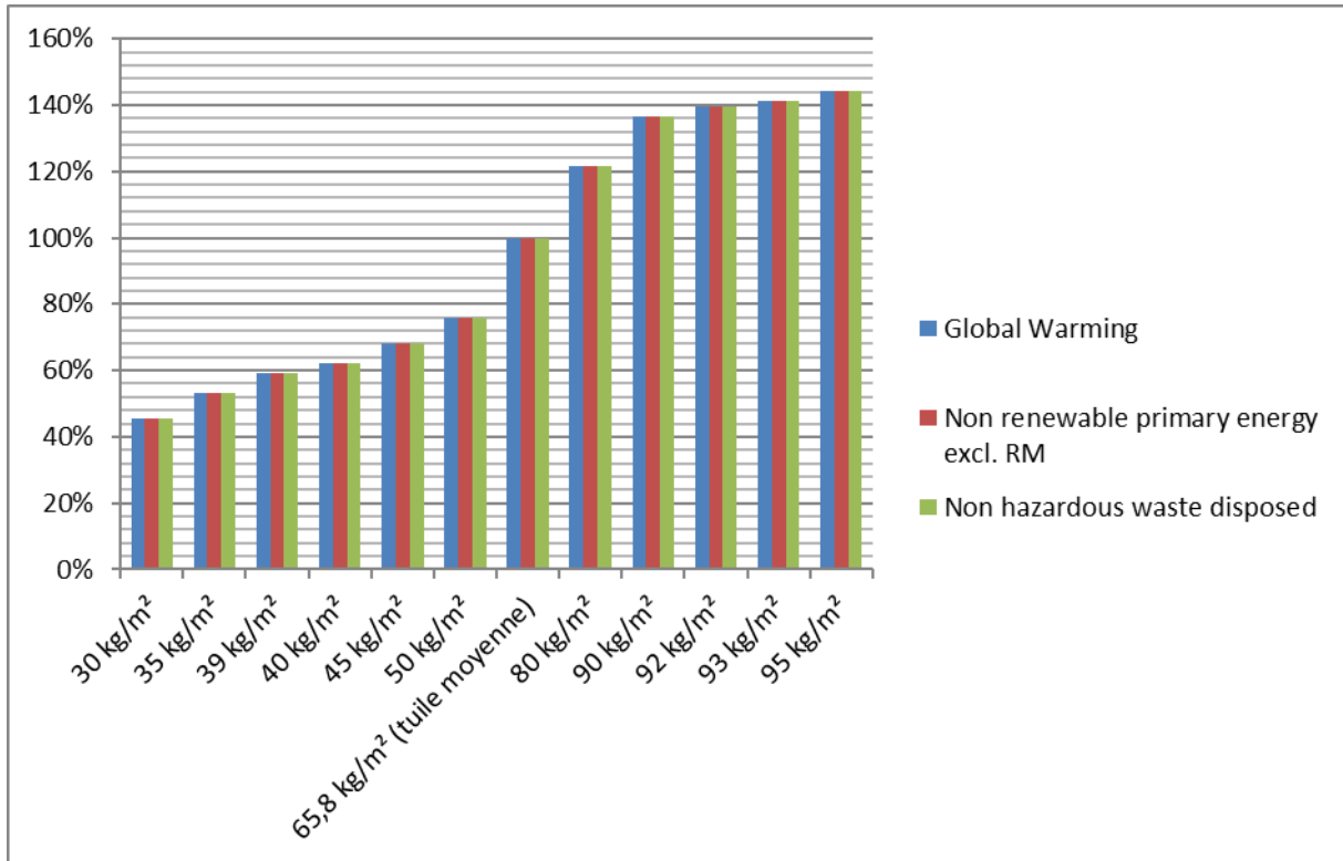
Graphique illustrant la variabilité des résultats d'impacts environnementaux sur 3 indicateurs en fonction de la variation de la masse de tuiles au mètre carré
