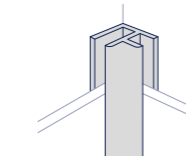
Angle universel en aluminium (ref 06440001) Angle universel noir en aluminium (ref 06440002)
