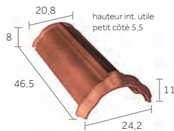
Arêtier de 40° à emboîtement (2,5 au ml)
