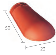
Arêteur d'about pour faîtière/arêteur conique de 40
