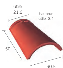
Faîtière/arêteur conique de 50 (2,4 au ml)
