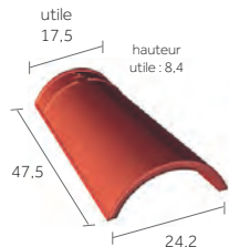
Faîtière/arêteur conique de 40 (2,5 au ml)
