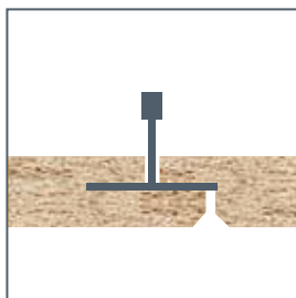
BORDS CACHÉS DÉMONTABLES (CD)
